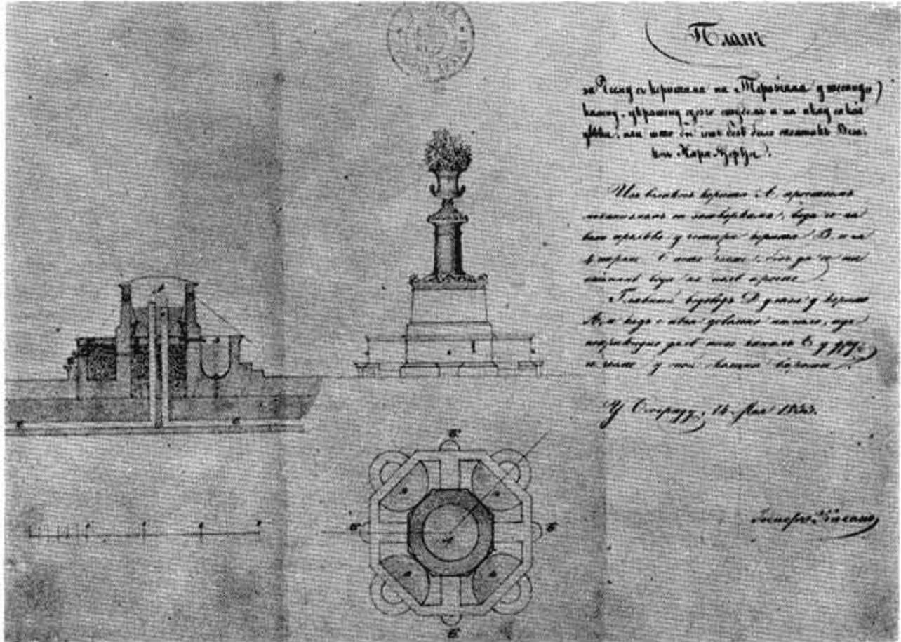
Сл. 1 — Први план Теразиске чесме Јосифа Касана
