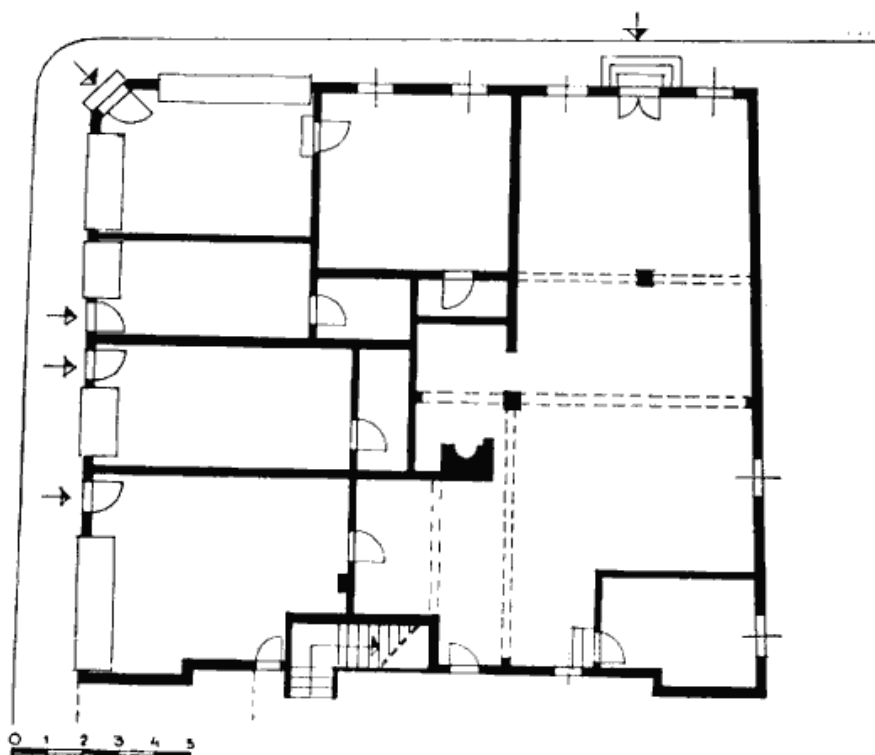
Сл. 3 — Основа приземља са дућанима према Бранковој улици и једним већим магацином
