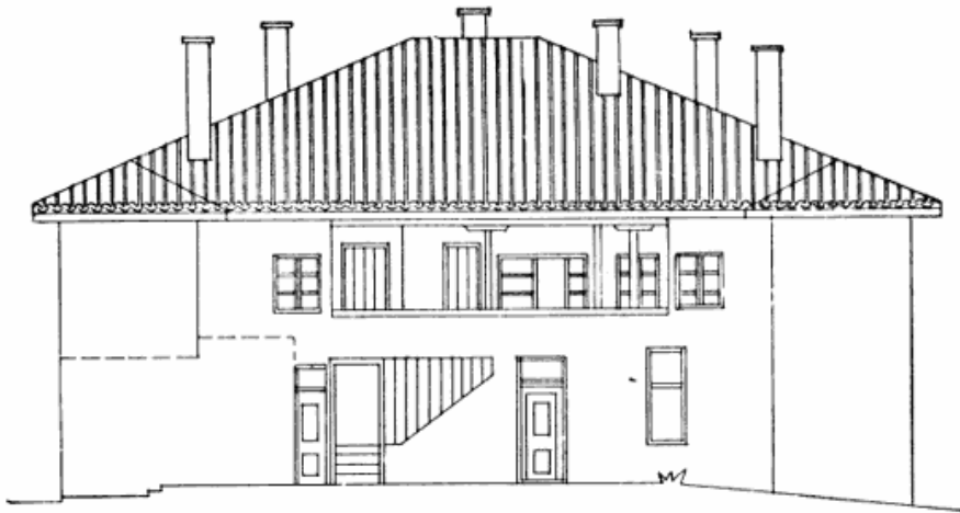
Сл. 4. — Изглед фасаде према дворишту са дивананом у горњем делу и видљивим степеништем. Цело решење је, и ако скромно, ипак скоро монументално, нарочито кад се апстрахују накнадно импровизовани отвори у приземљу
