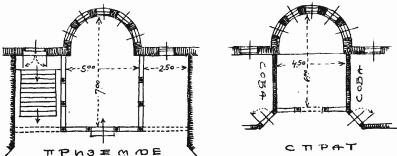
Сл. 1 — Основе двеју диван'ана у конаку кнегиње Љубице
