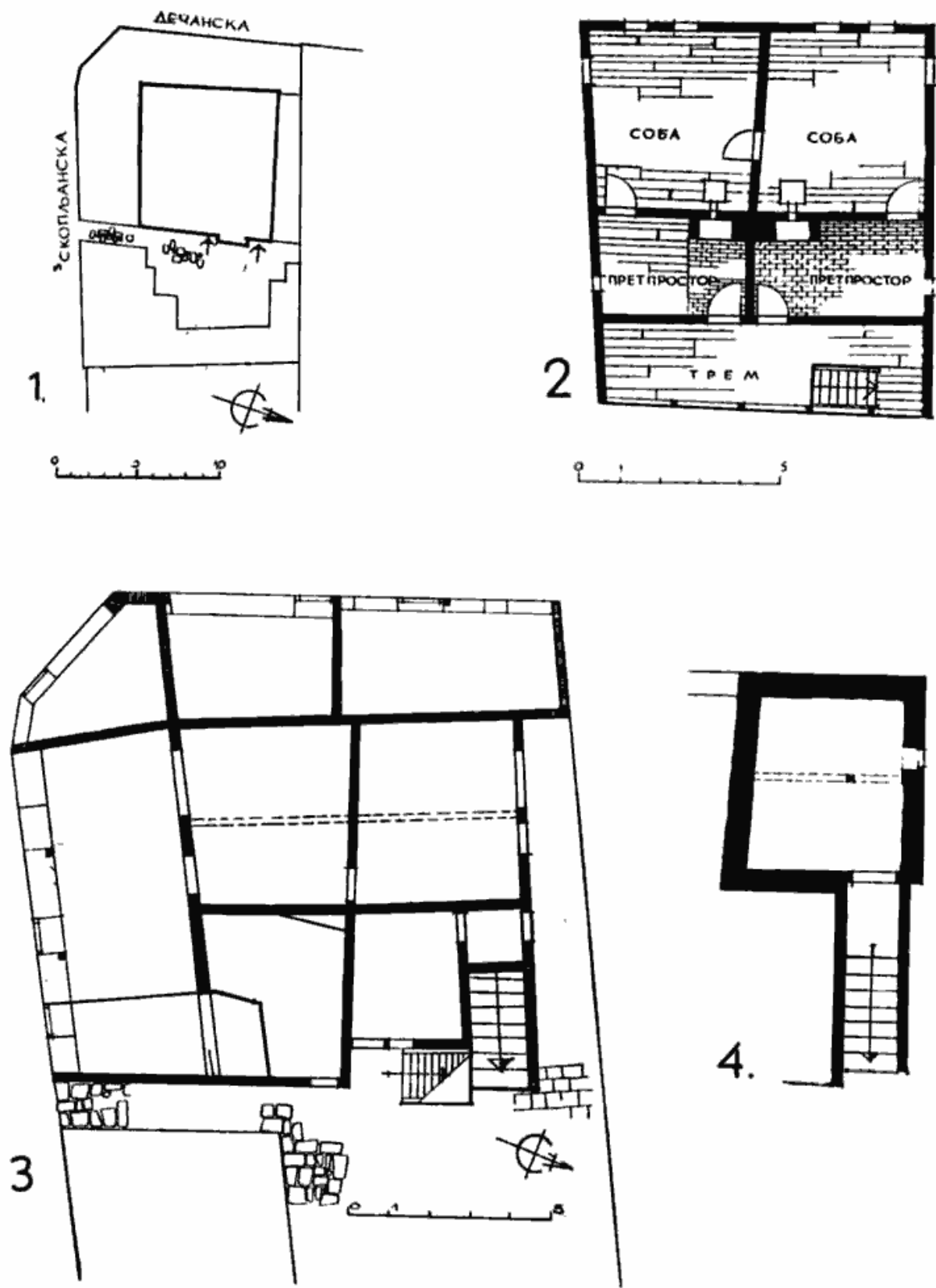
Сл. 2 — Стара кућа у Нушићевој улици: 1. Ситуација; 2. Основа спрата; 3. Основа приземља; 4. Основа подрума
